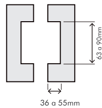
VIDRO | VIDRO (Rasgo)
